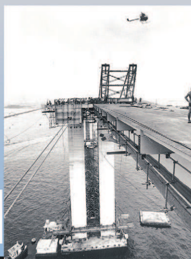
Fotos mostram a construção e a inauguração da Ponte Presidente Costa e Silva mais conhecida como Ponte Rio-Niterói.
